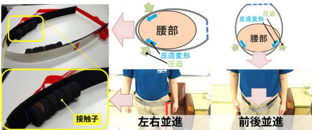
腰部ハンガー反射による並進力提示の様子
